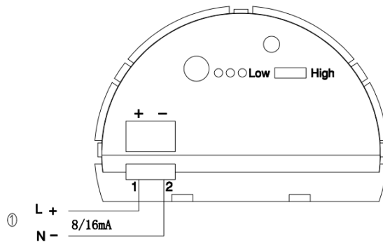
图7 二线制输出方式
