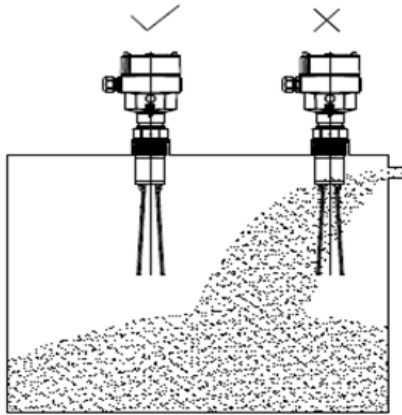
图 4 避免入料口的安装示意图
