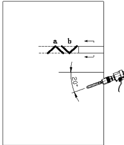
图 2 水平安装示意图
