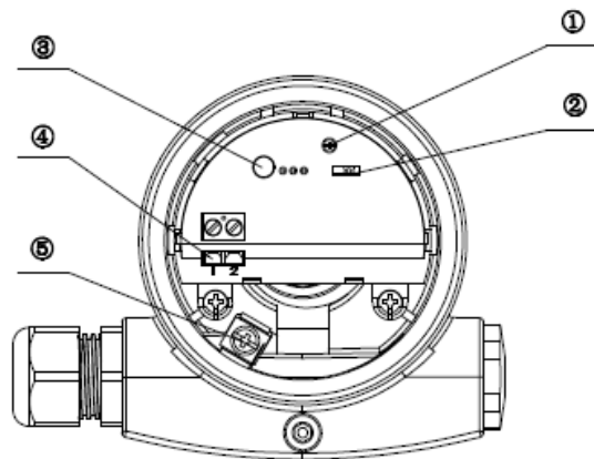
图9 二线制输出方式
