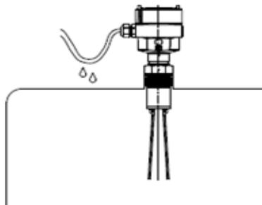
图 5 防潮安装
