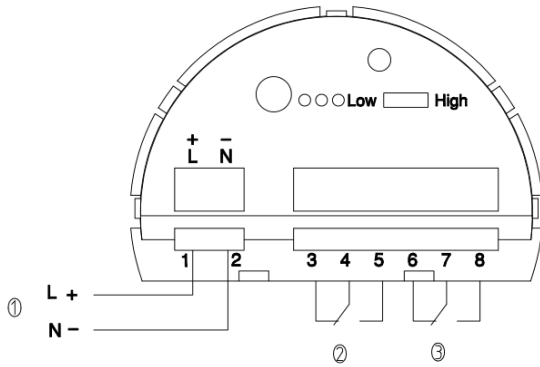
图6 继电器输出方式
